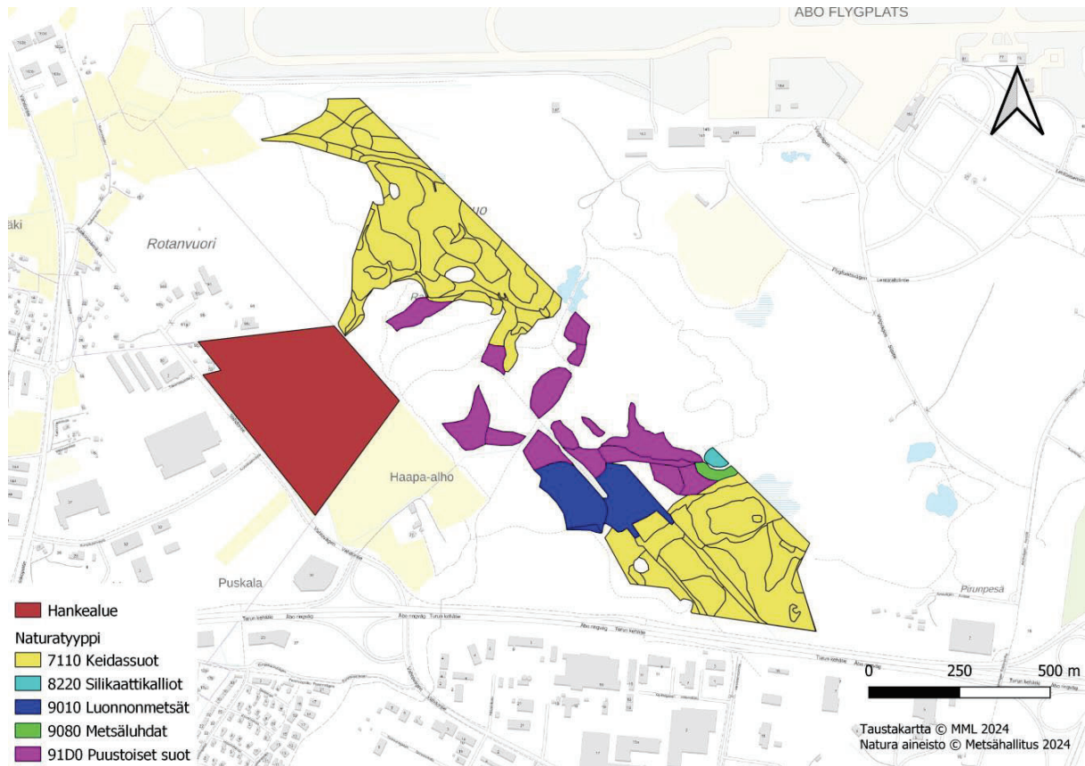
Kuva 7. Pomponrahkan Natura-luontotyypit (Metsähallitus tietopyyntö 2024).
