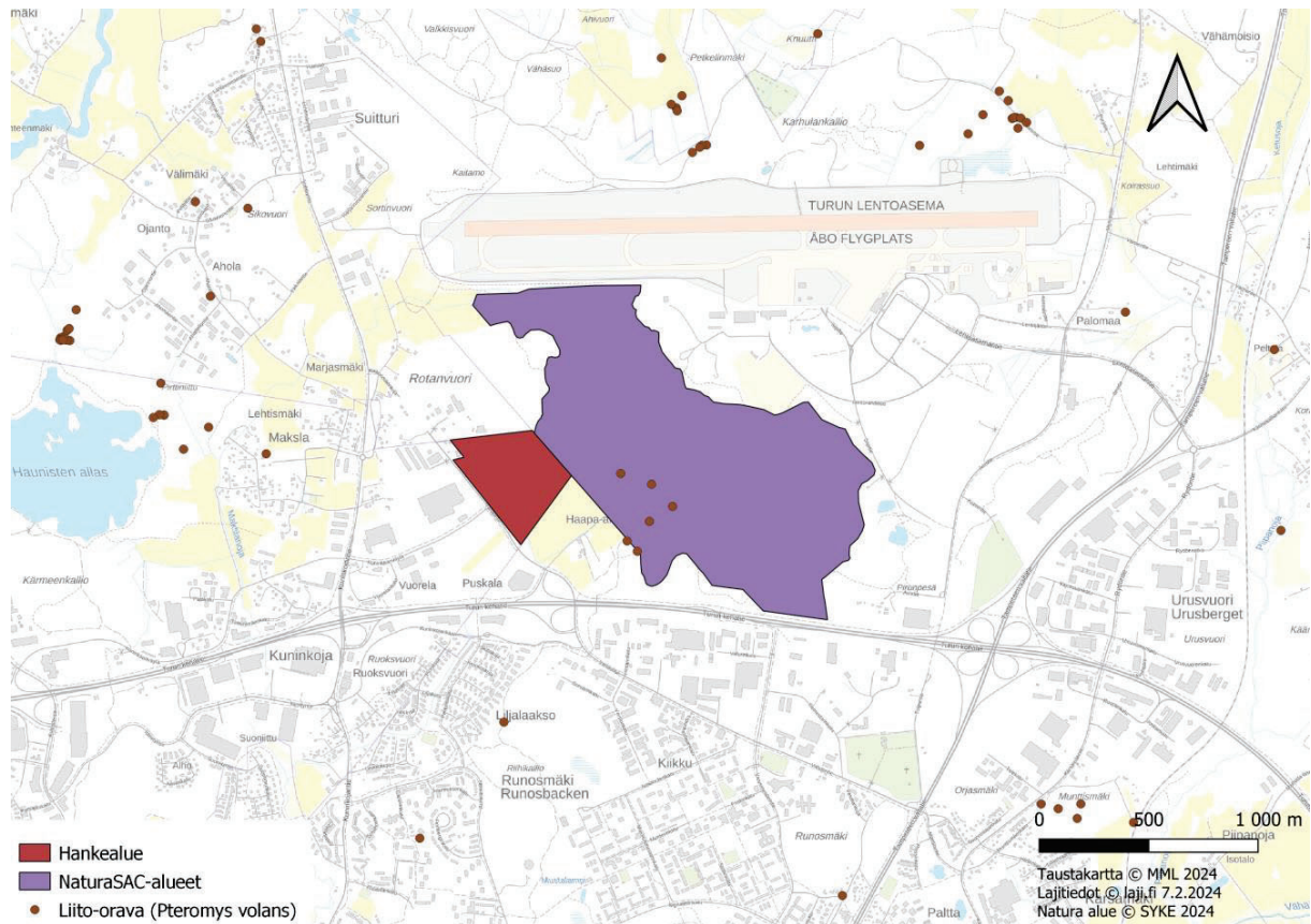
Kuva 8. Liito-oravahavainnot hankealueen läheisyydessä ja Pomponrahkan Natura-alueella (Suomen lajitietokeskus tietopyyntö 7.2.2024).
