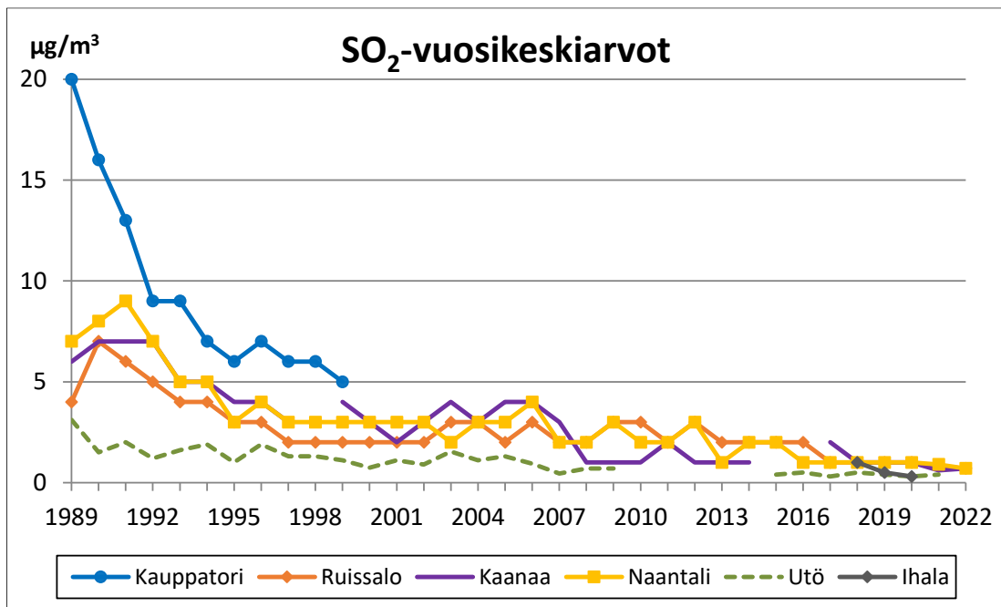
Kuva 11. Rikkidioksidin vuosikeskiarvojen kehitys vuosina 1989–2022
